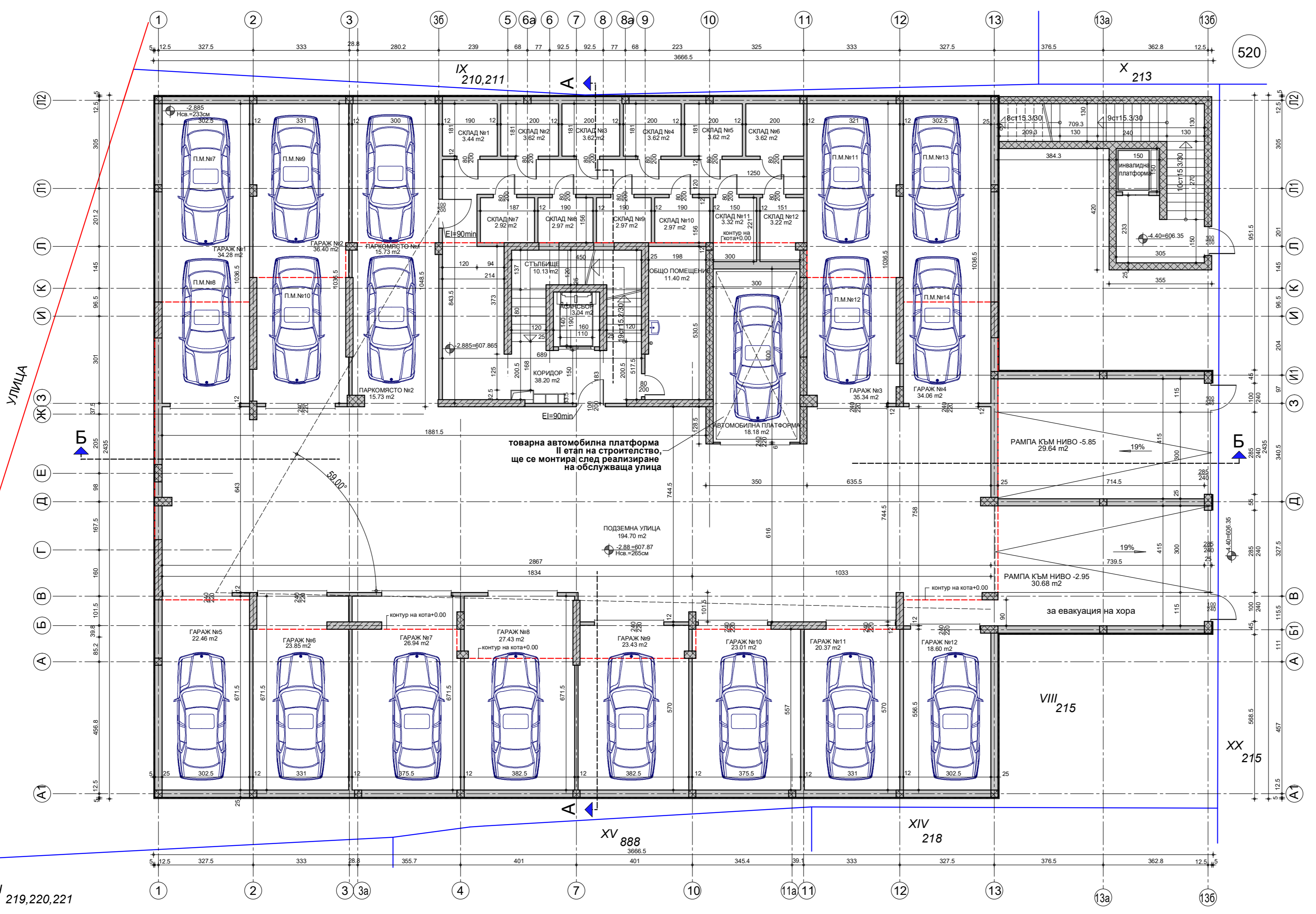
ПЛАН КОТА -2.88 М 1:100
