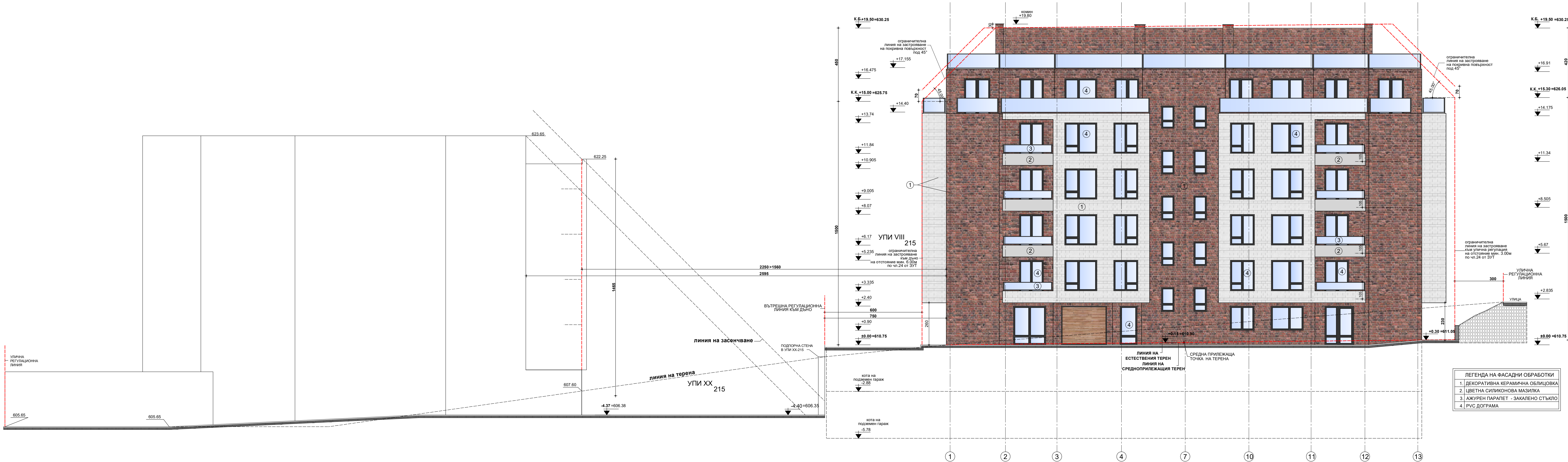
ФАСАДА "СЕВЕРОИЗТОК" М 1:100
